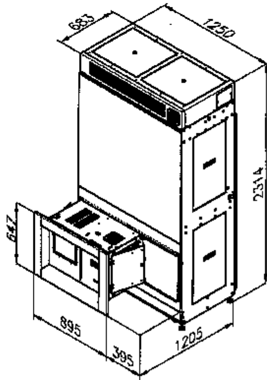
INGOMBRI VIDEODISTRIBUTORE
