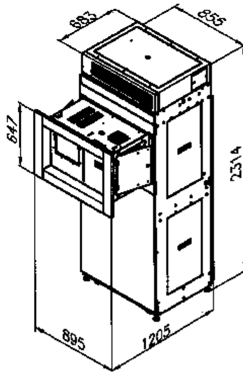
INGOMBRI VIDEODISTRIBUTORE
