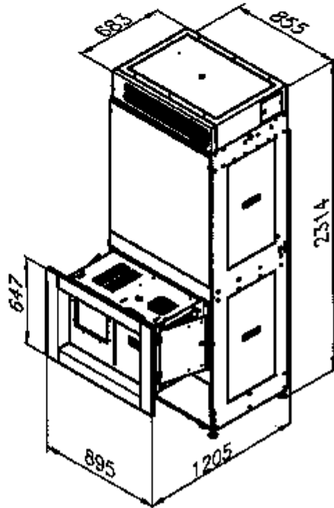
INGOMBRI VIDEODISTRIBUTORE
