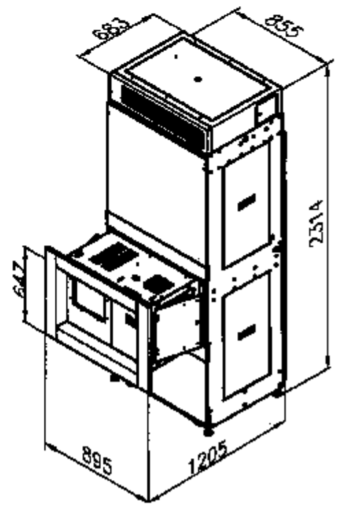
INGOMBRI VIDEODISTRIBUTORE
