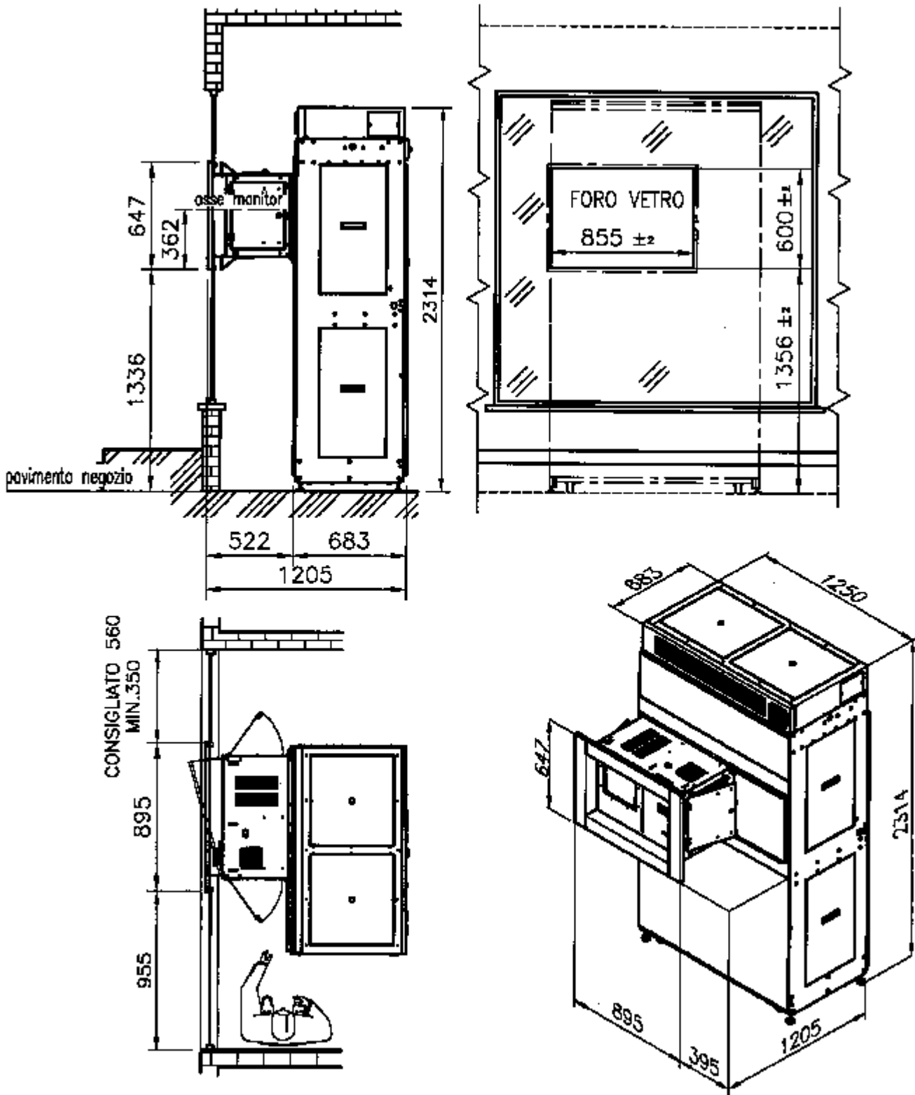
INGOMBRI VIDEODISTRIBUTORE
