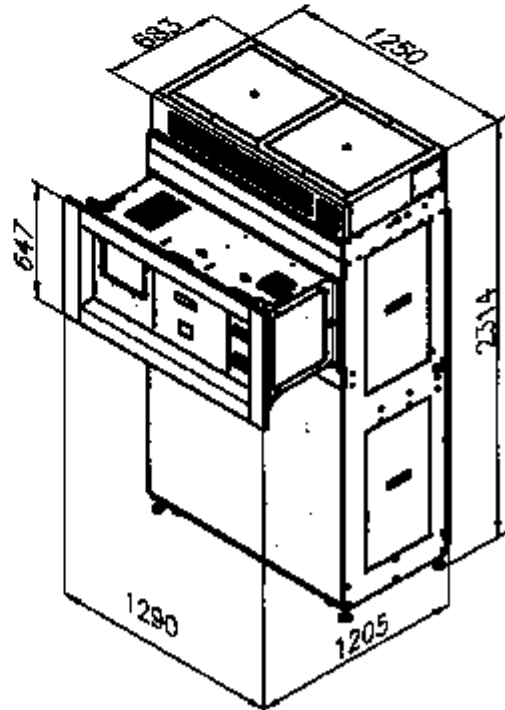
INGOMBRI VIDEODISTRIBUTORE
